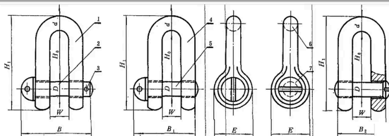
图 1 1—ZA 本体; 2—光直销; 3—开口销; 4—ZB 本体; 5—螺纹销; 6—ZC 本体; 7—槽孔销
