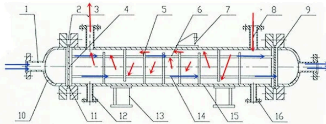
1、管箱 2、螺栓 3、螺母 4、管板 5、折流板 6、换热管 7、耳架 8、排气口 9、设备法兰 10、封头 11、垫片 12、排液口 13、支座 14、拉杆 15、筒体 16壳程接管
