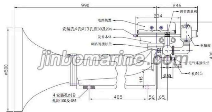
图(五)WD-2A型气笛外形尺寸和安装尺寸
