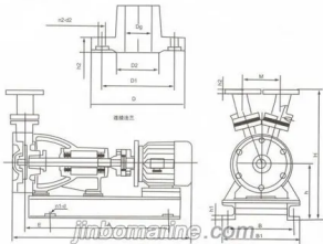
安装尺寸图 Installation Dimensions
