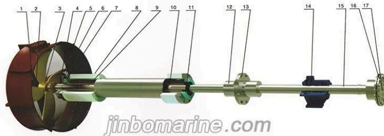
船舶主推进系统——轴系示意图 The basic marine main propulsion system—shaft sketch map
