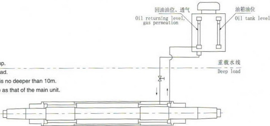
艉轴润滑系统原理
