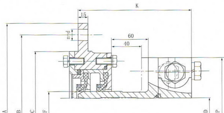
JQ/CS 49前密封装置 JQ/CS 49 forward sealing apparatus
